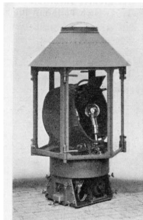
Abb. 8. Drehfeuer, Siemens-Schuckert Type DF.
