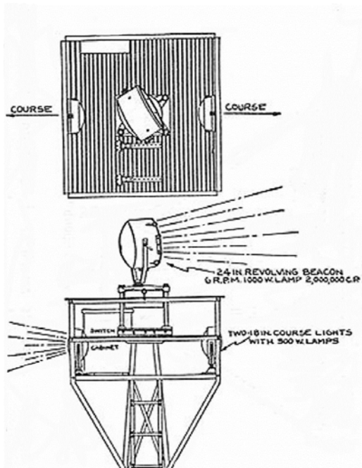
Esquema instalación aerofaro de ruta.
