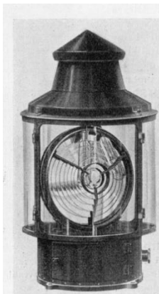
Abb. 13. Pintsch-Drehlinseleuchte DL 150, Lichtstärke 1,7 Mill. HK.
