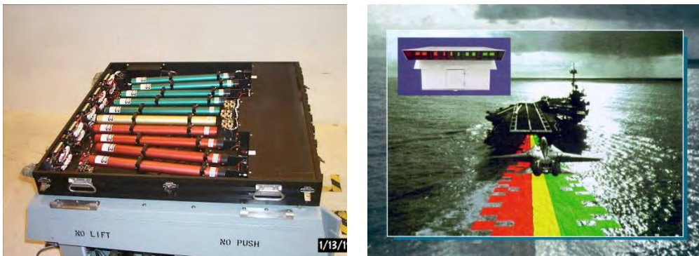
Sistema de guiado Láser. LRLS. a) Unidad con 10 láser. b) Recreación de la visualización de un LRLS.
