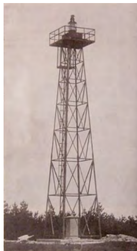
Aerofaro de Hellenendoorn. Torre celosía de acero de 17 m de alto. 1930
